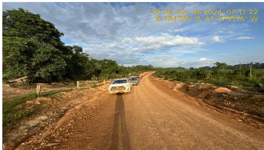
Serviços de Recomposição do Revestimento Primário (encascalhamento) e saída d'água (bigode).
