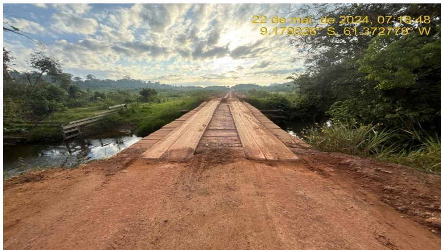
Serviços de Reforma de ponte de madeira (troca de rodeiro e assoalho).
